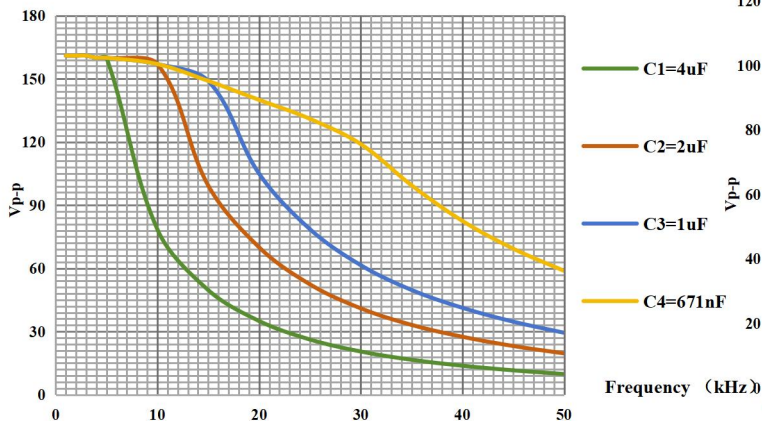
ATA-308C 容性负载曲线图
