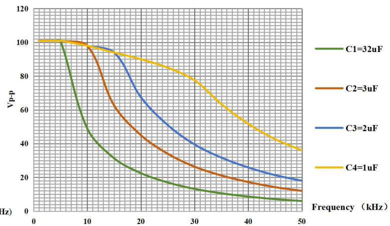
ATA-304C 容性负载曲线图
