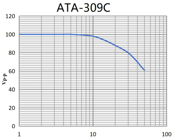
幅频特性 (最大输出电压 Vp-p)
