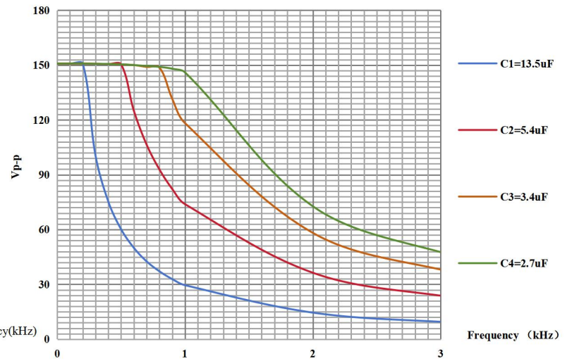
ATA-P0102 容性负载曲线图
