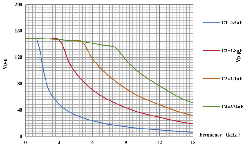
ATA-P1005 容性负载曲线图
