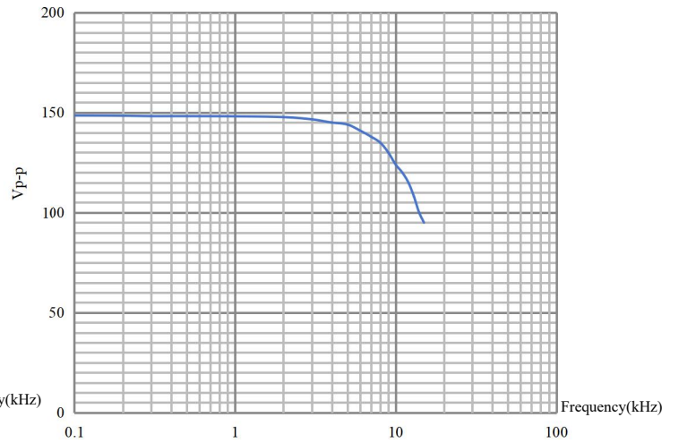
幅频特性 (最大输出电压 Vp-p)
