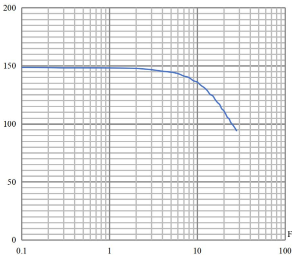
幅频特性 (最大输出电压 Vp-p)
