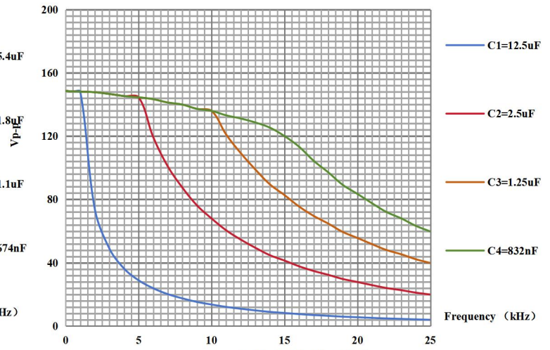
ATA-P2010 容性负载曲线图
