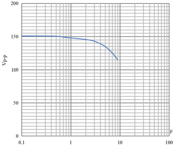
幅频特性 (最大输出电压 Vp-p)
