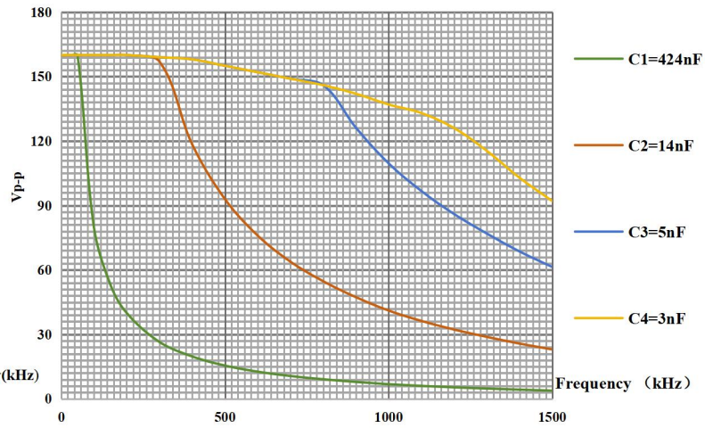
ATA-4011C 容性负载曲线图
