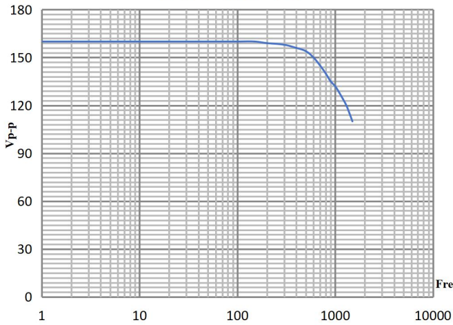
幅频特性 (最大输出电压 Vp-p)
