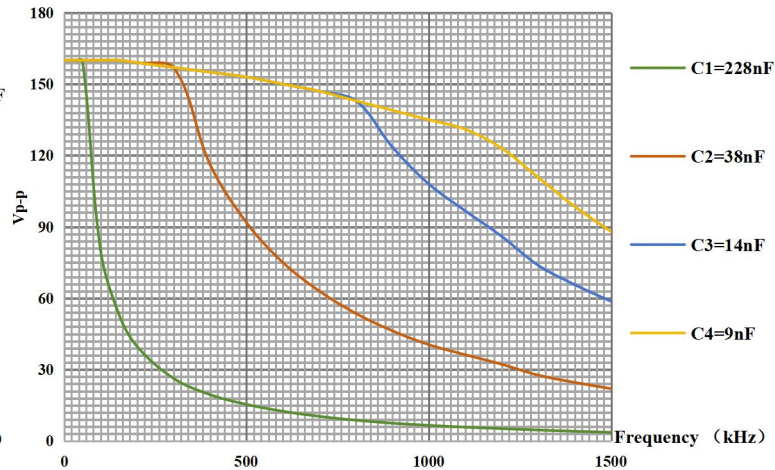
ATA-4014C 容性负载曲线图
