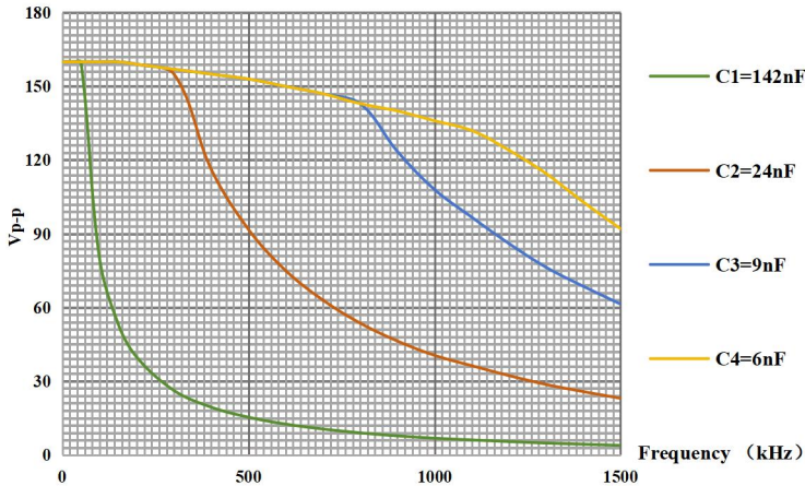
ATA-4012C 容性负载曲线图
