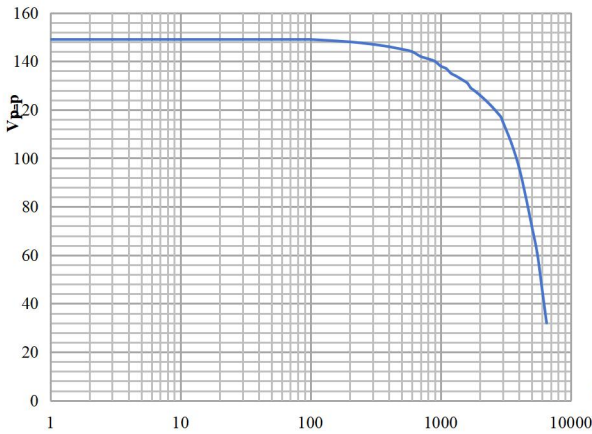
幅频特性 (最大输出电压 Vp-p)
