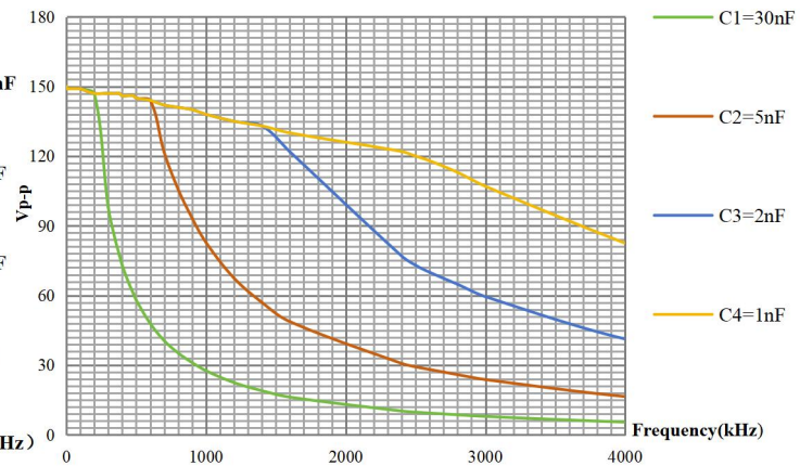
ATA-4315 容性负载曲线图
