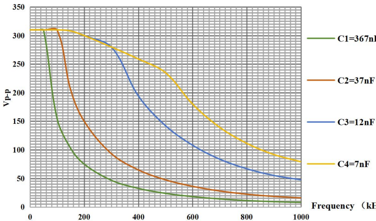
ATA-4052C 容性负载曲线图
