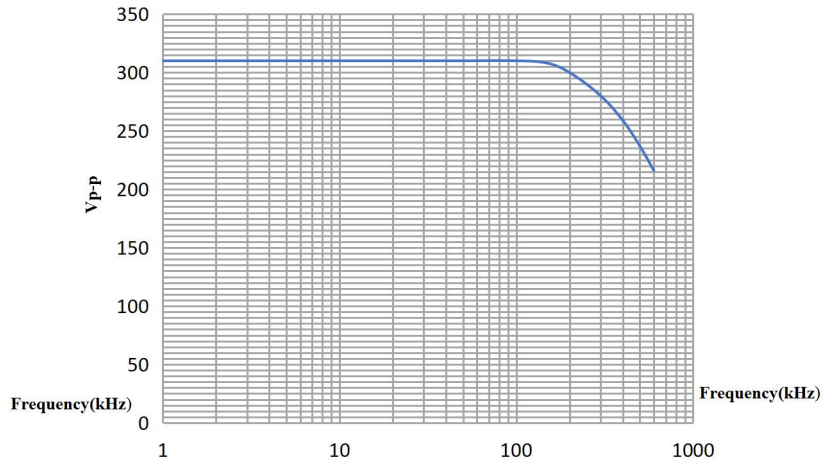
幅频特性 (最大输出电压 Vp-p)
