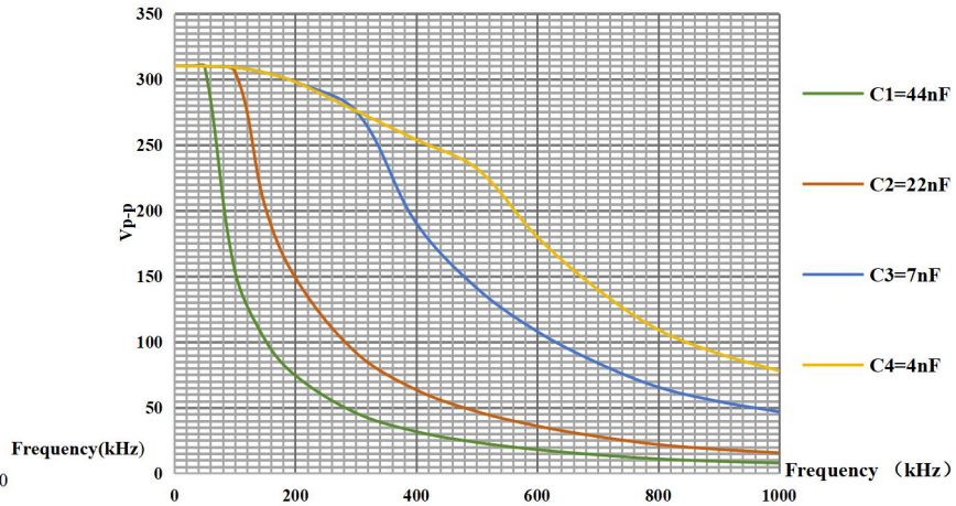
ATA-4051C 容性负载曲线图
